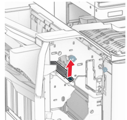
9 以逆時鐘方向轉動旋鈕 R3，然後取出 1 號出紙槽中的夾紙。
